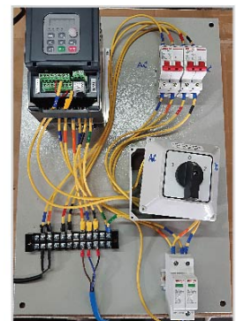
ตัวอย่างการต่อสายไฟ แผงวงจร
