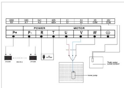
ตัวอย่างการต่อสายภายในกล่อง AC/DC INVERTER
