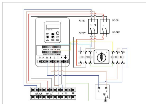
ตัวอย่างการต่อวงจรสายไฟ เข้ากับกล่อง AC/DC INVERTER
